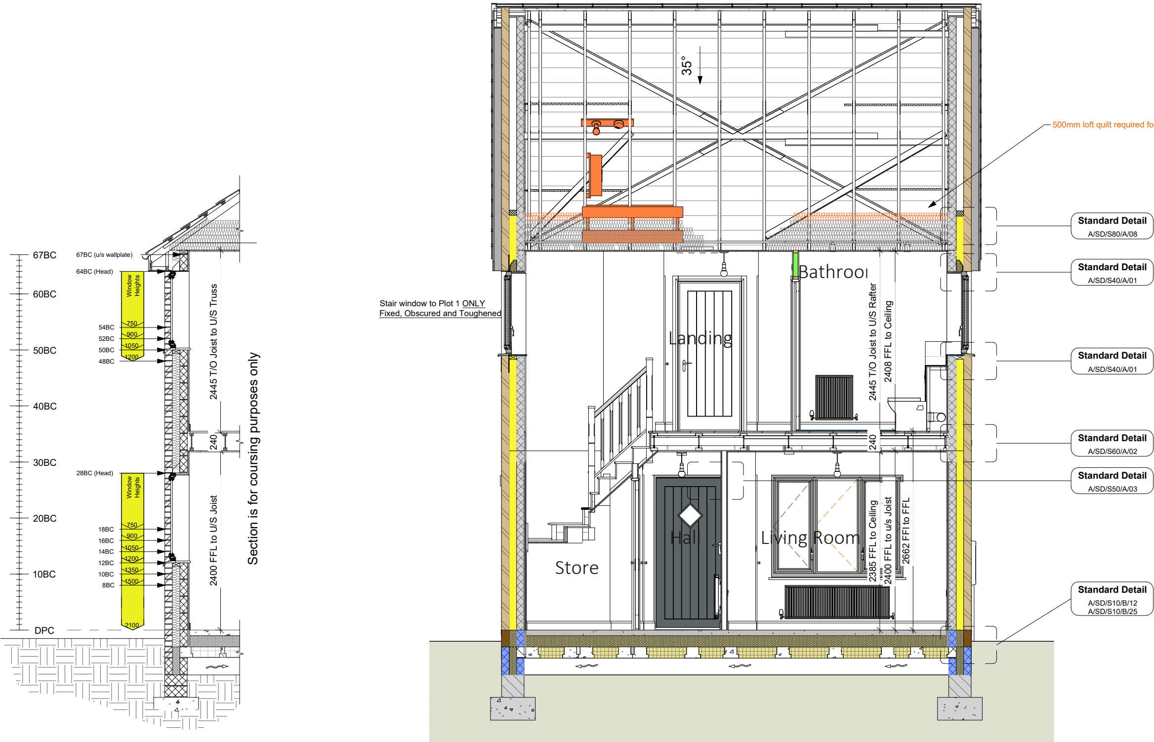
C Section D - D 1 : 50
